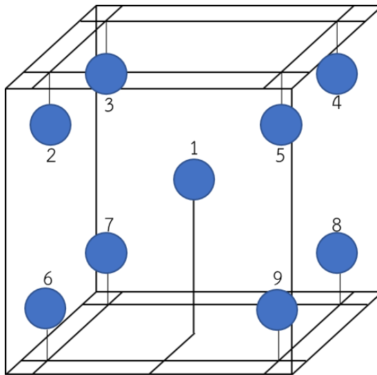
รูปที่ 4.26 ตำแหน่งการติดตั้งอุปกรณ์ตรวจวัดอุณหภูมิการทดสอบการกระจายความเย็นภายในตู้ห้องเย็น
