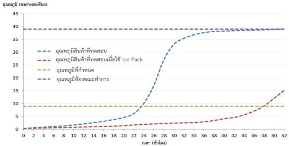
รูปที่ 4.4 ตัวอย่างแสดงผลการทดสอบประสิทธิภาพวัสดุกักเก็บความเย็นกับสินค้าแช่เย็น
