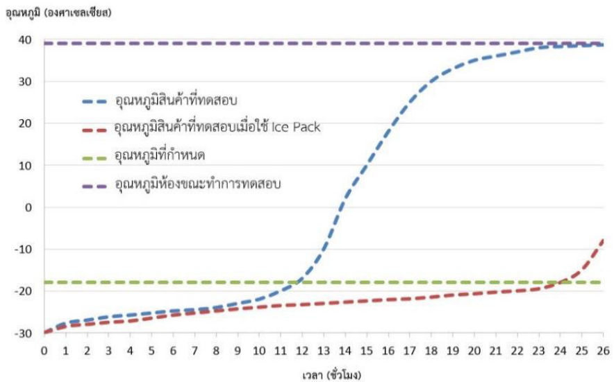
รูปที่ 4.5 ตัวอย่างแสดงผลการทดสอบประสิทธิภาพวัสดุกักเก็บความเย็นกับสินค้าแช่แข็ง
